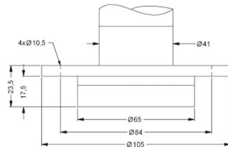
Flansch DRD 5
