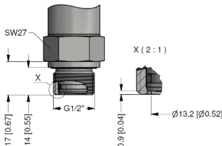
G1/2" frontbündig DIN 3852 (0,1 bar ≤ p N ≤ 40 bar)
